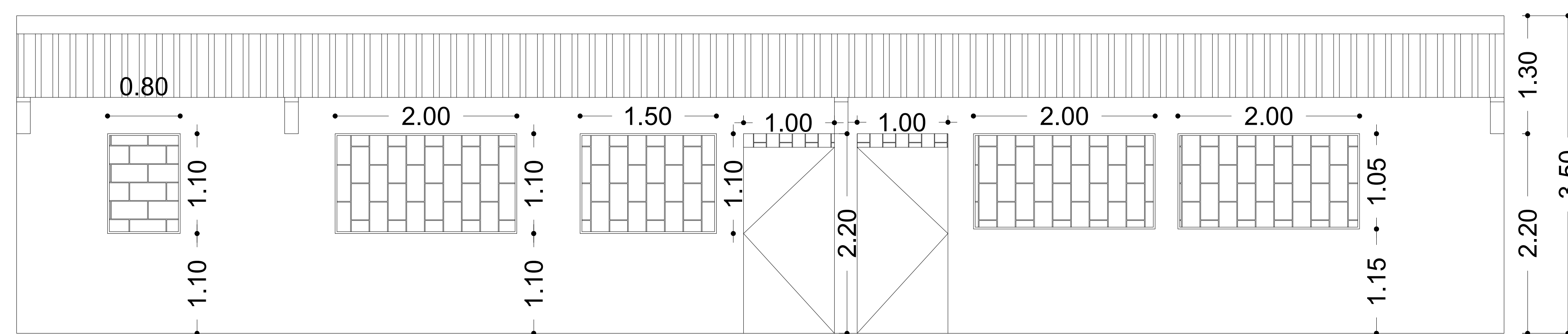
FACHADA PRINCIPAL EDIFICIO 1
