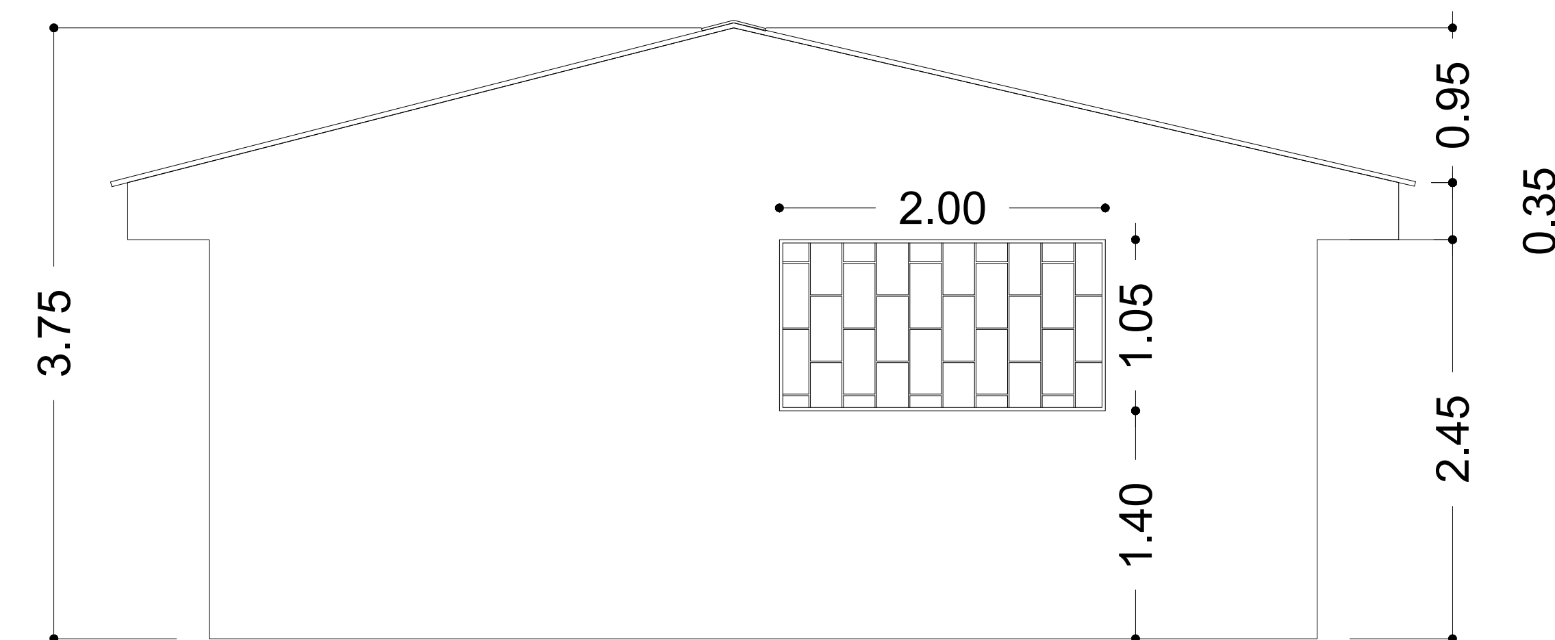
FACHADA LATERAL DERECHA EDIFICIO 1
